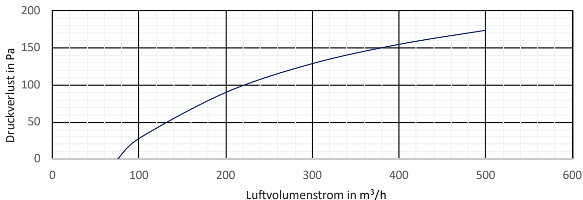
Druckverlust-diagramm F7 für Baugröße 100, 125 und 160
