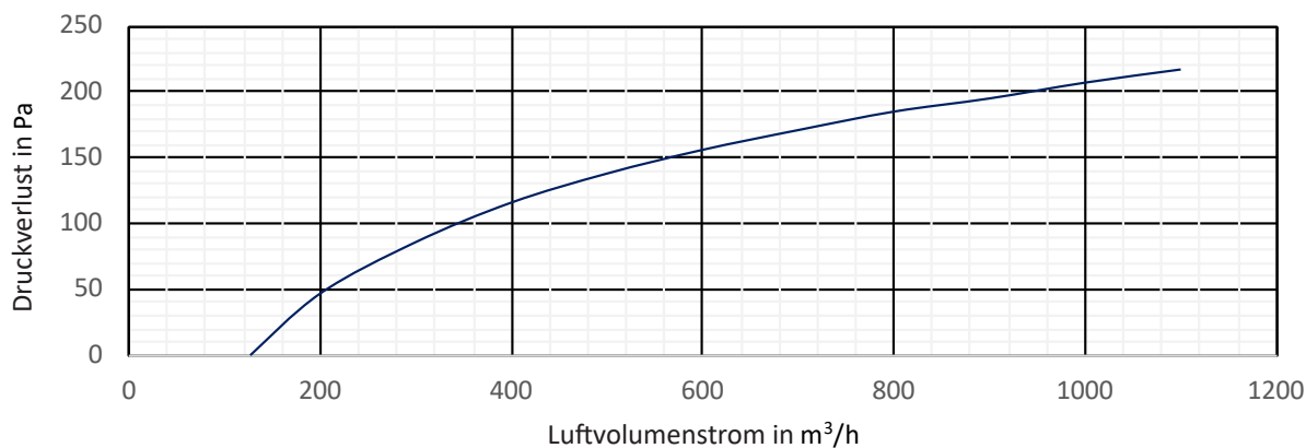
Druckverlust-diagramm F7 für Baugröße 200 und 250
