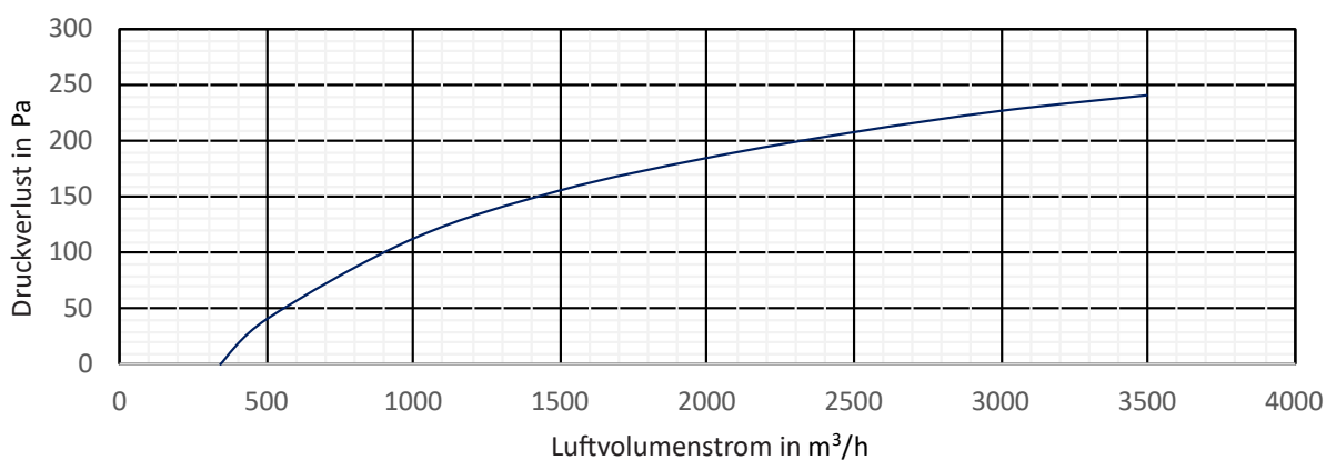
Druckverlust-diagramm F7 für Baugröße 315, 355 und 400
