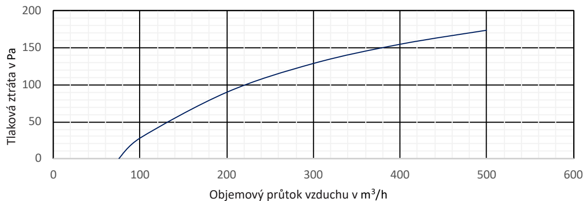
Diagram tlakové ztráty F7 pro velikosti 100, 125 a 160
