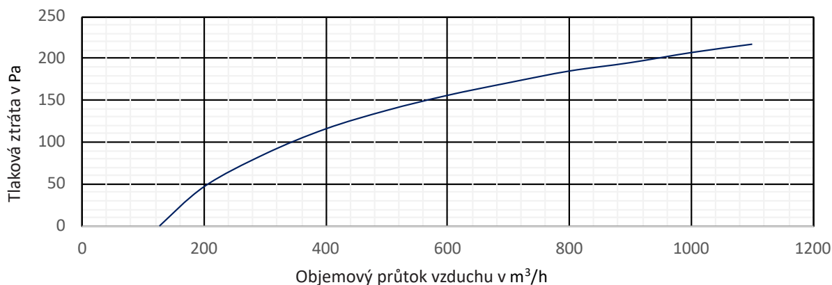
Diagram tlakové ztráty F7 pro velikosti 200 a 250
