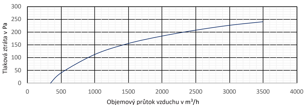
Diagram tlakové ztráty F7 pro velikosti 315, 355 a 400
