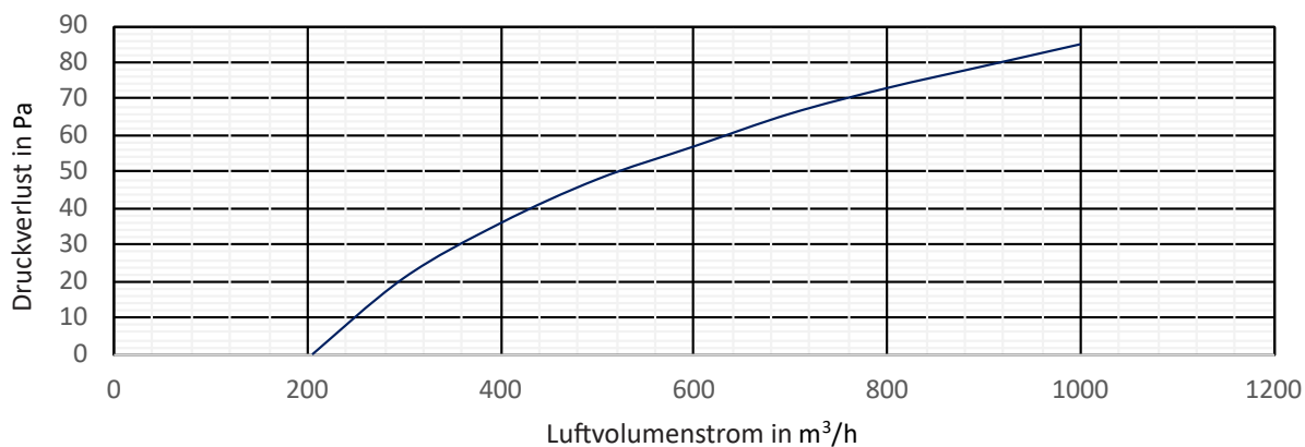
Druckverlust-diagramm G4 für Baugröße 200 und 250
