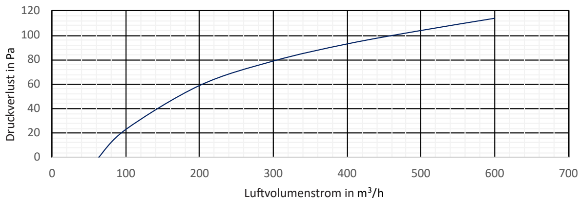
Druckverlust-diagramm G4 für Baugröße 100, 125 und 160
