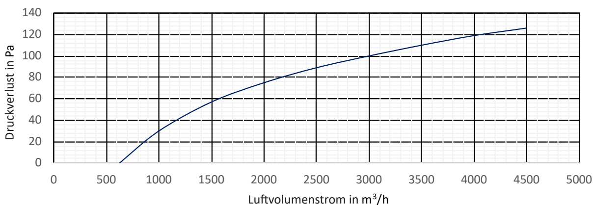
Druckverlust-diagramm G4 für Baugröße 315, 355 und 400
