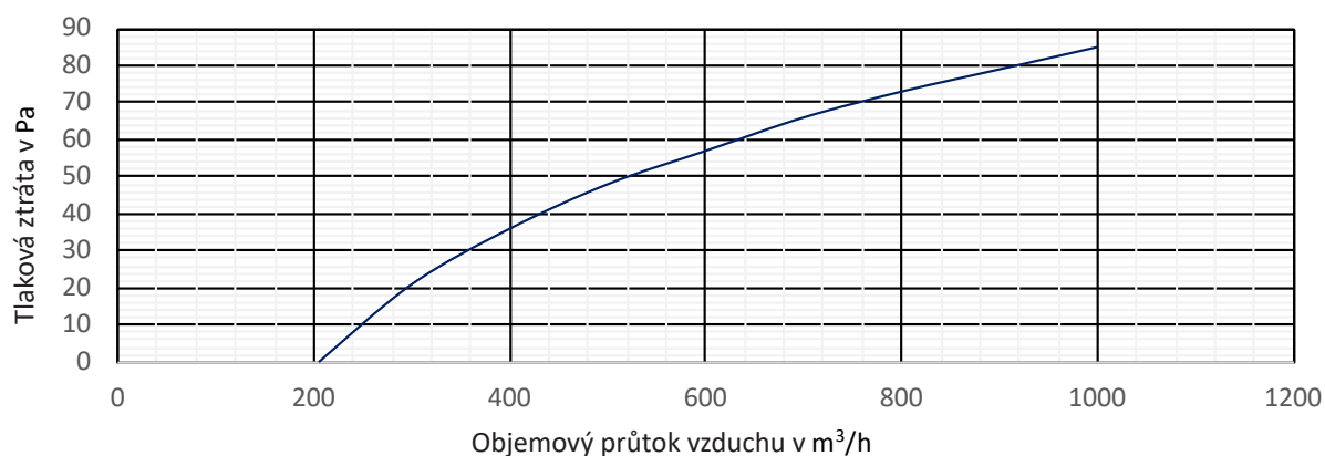
Diagram tlakové ztráty G4 pro velikosti 200 a 250
