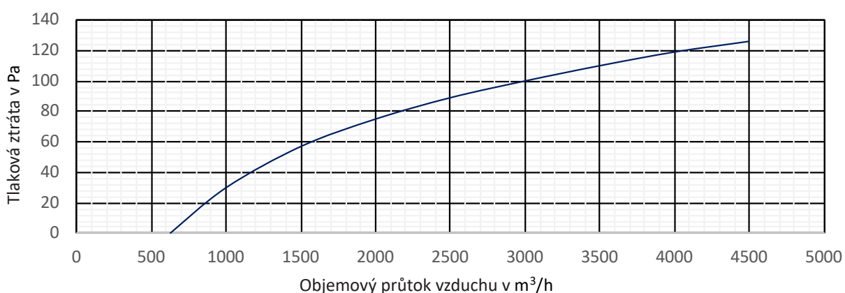
Diagram tlakové ztráty G4 pro velikosti 315, 355 a 400
