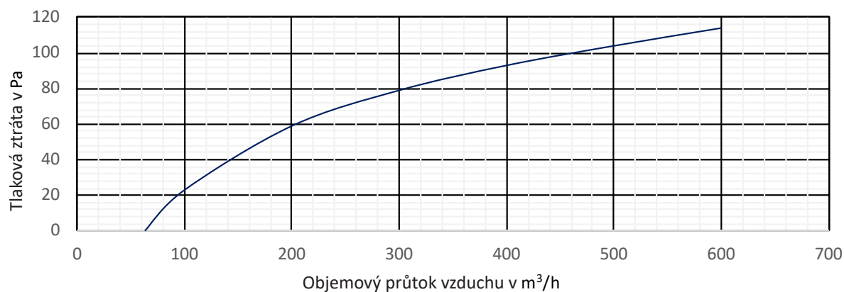
Diagram tlakové ztráty G4 pro velikosti 100, 125 a 160
