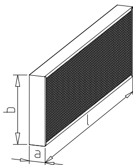
Kulisa tlumiče hluku
