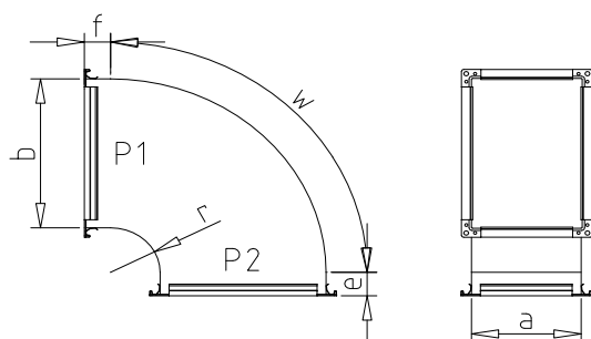
20 - Oblouk symetrický
