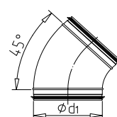
OK-Oblouk lisovaný 45°
