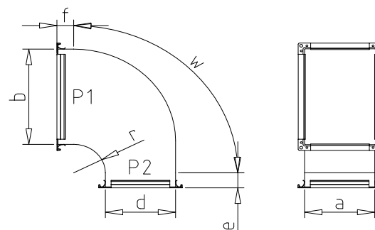
21 - Oblouk asymetrický
