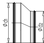
OK-Přechod asymetrický
