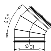
OK-Oblouk segmentový 45°
