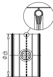
OK-Kruhová klapka těsná
