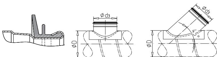
OK-Sedlová odbočka 90° OK-Sedlová odbočka 45°
