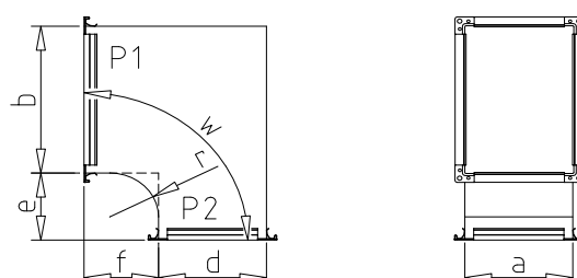
31 - Koleno asymetrické
