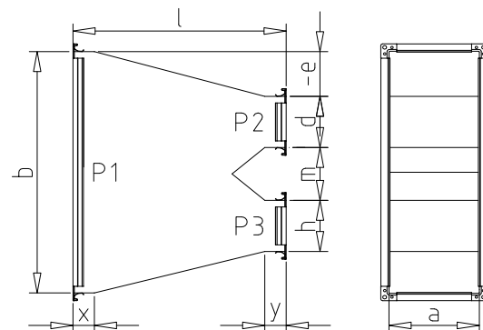
80 - Kalhotový kus symetrický
