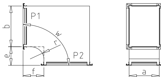
30 - Koleno symetrické
