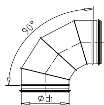
OK-Oblouk segmentový 90°
