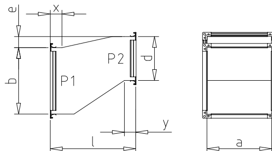
61 - Odskok asymetrický
