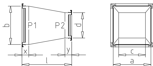
40 - Přejchod symetrický
