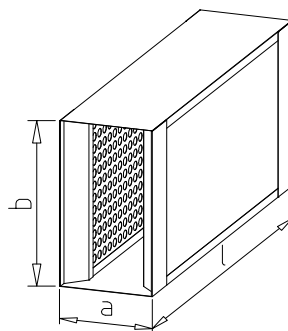
Schalldämpferzelle mit Lochblech
