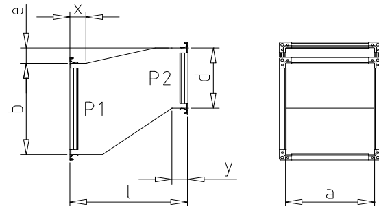
61 - Etage asymmetrisch
