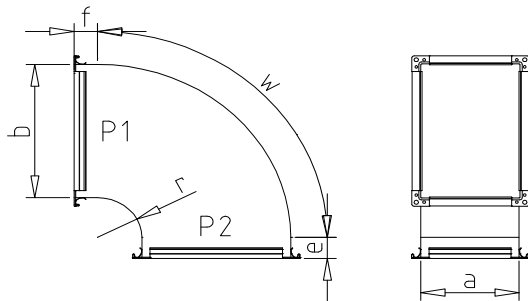
20 - Bogen symmetrisch
