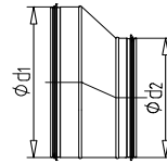
OK-Reduzierung asymmetrisch
