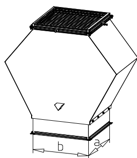
Deflektorhaube eckig
