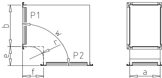
30 - Winkel symmetrisch
