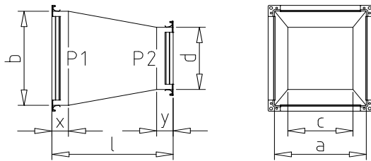
40 - Übergang symmetrisch
