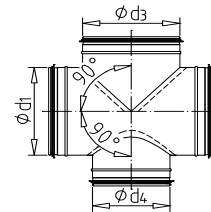
OK-Kreuzstück 90°
