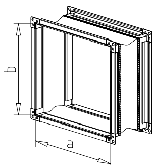
Segeltuchstutzen
