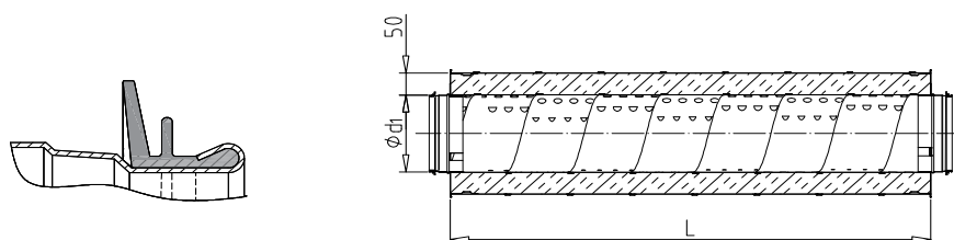
OK-Rohrschalldämpfer OK-Rohrschalldämpfer OK-Rohrschalldämpfer OK-Rohrschalldämpfer L=600 / 50 L=900 / 50 L=1200 / 50 L=1500 / 50
