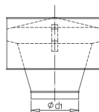
CAGI Haube
