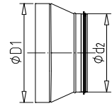
OK-Reduzierung symmetrisch M/N
