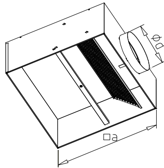
Anschlusskasten Anschlusskasten Zuluft Abluft
