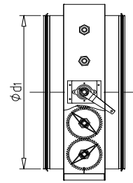
OK-Rechteckige Klappe mit rundem Anschluss
