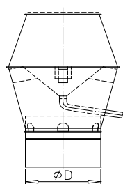
Deflektorhaube
