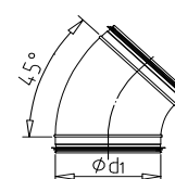
OK-Oblouk lisovaný 45°
