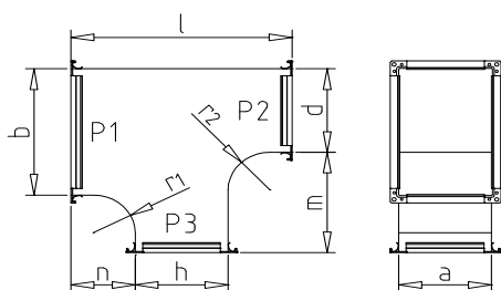
70 - T-kus symetrický
