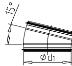
OK-Oblouk lisovaný 15°
