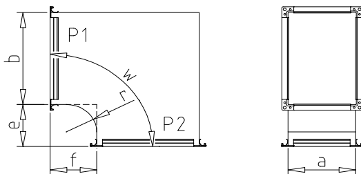
30 - Koleno symetrické
