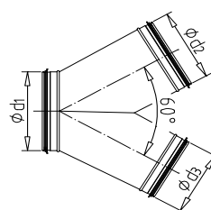
OK-Rozbočka symetrická 60°
