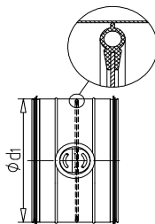
OK-Kruhává klapka těsná
