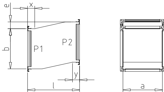
60 - Odskok symetrický
