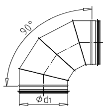
OK-Oblouk segmentový 90°
