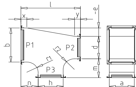
71 - T-kus asymetrický
