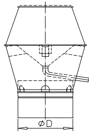
Výfuková hlavice
