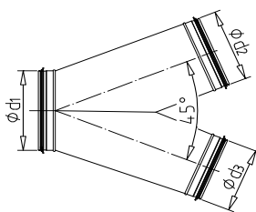
OK-Rozbočka symetrická 45°
