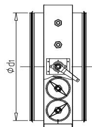
OK-Hranatá klapka s kruhovým připojením
