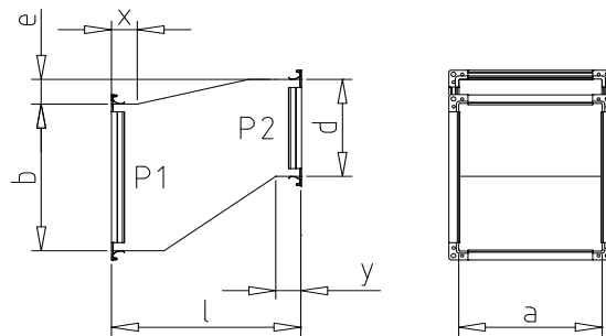
61 - Odskok asymetrický
